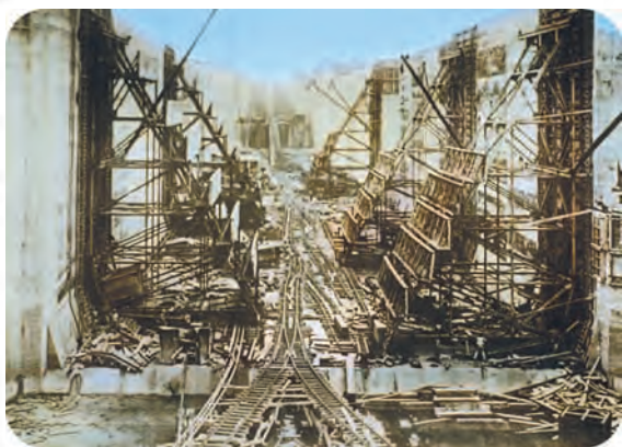
CANAL DE PANAMÁ — COMPUERTA DE GATÚN ARRIBA
