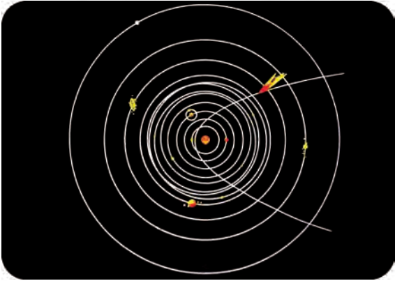
NUESTRO SISTEMA PLANETARIO
